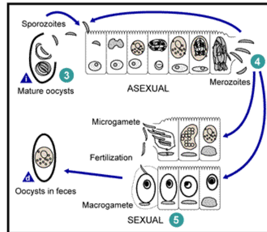
Cycle d' Isospora belli
